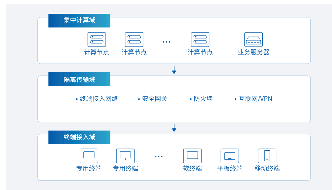
▲ 系单数据中心部署图
